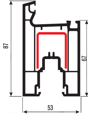
PRSY02 Kanat Profili Sash Profile DS-01
