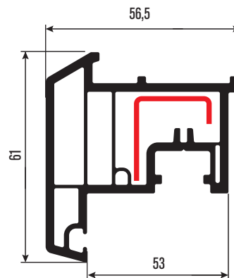
PRFS13 Hareketli Orta Kayıt Stump (Overhang) DS-13
