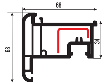
PR7113 Hareketli Orta Kayıt Stump (Overhang) DS-12
