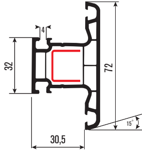
PRS603B Orta Kayıt Profili Mullion Profile
