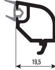
PRVN17 Tek Cam Çıtası 20mm Double Glazing Bead
