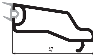
PR7114 Tek Cam Çıtası Single Glazing Bead
