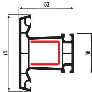
PRFS03 Orta Kayıt Profili Mullion Profile DS-3
