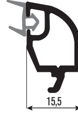
PRVN19 24mm Çift Cam Çıtası 20mm Glazing Bead
