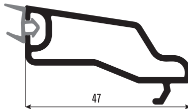
PR7114 Tek Cam Çıtası Single Glazing Bead
