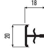
PRTS24 İnce Bağ Profili Coupling
