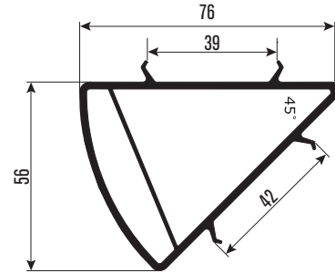
PR7129 45° Köşe Adaptörü 45° Corner Adapter
