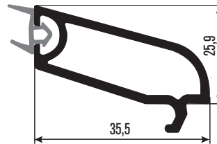
PRVN14 Tek Cam Çıtası Single Glazing Bead
