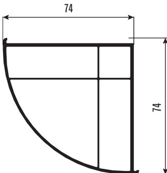
PR7130 90° Köşe Adaptörü 90° Corner Adapter
