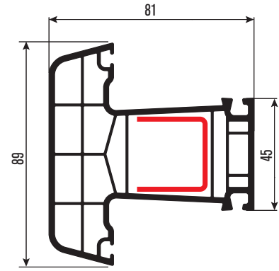
PRGR03 Orta Kayıt Profili Mullion Profile DS-1
