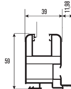
PRPJ78 Geçmeli Yan dikme Pass Side Strut
