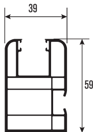
PRPJ91 59 mm Yan Dikme 59 mm Edge Pillar
