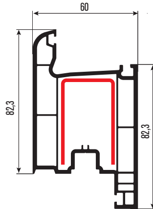
PRVN04 Kilitli Kapı Profili Door Sash Profile DS-8 DS-14
