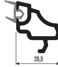
PR6018 Çift Cam Çıtası Double Glazing Bead
