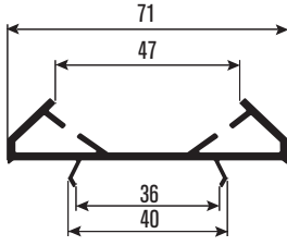
PR7127 Köşe Dönüş Adaptörü Adaptor To Turn Corner
