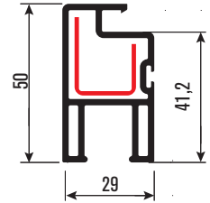
PRSY48 Sineklikli Kanat Profili Sash Fly Screen Profile
