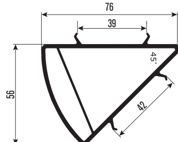
PR7129 45° Köşe Adaptörü 45° Corner Adapter
