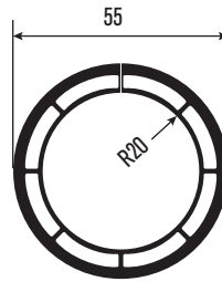
PRFS28 55 Boru 55 Pipe
