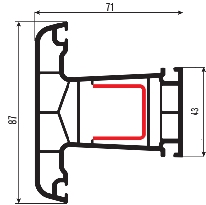
PRDR03 Orta Kayıt Profili Mullion Profile DS-2 DS-3
