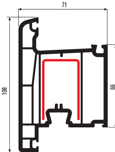
PR7105 Dışa Açılım Kapı Profili Outside Opening Door Sash Profile DS-8 DS-14
