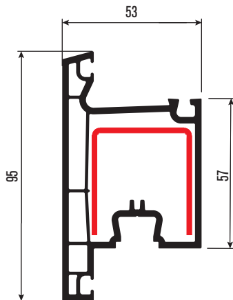
PRFS05 Dışa Açılım Kapı Profili Outside Opening Door Sash Profile DS-10
