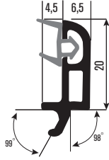
PRS621B Sürme 20 mm Çıta Sliding 20 mm Bead
