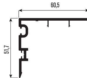
PRSY38 Sürme Kanat Adaptörü Sliding Sash Adaptor
