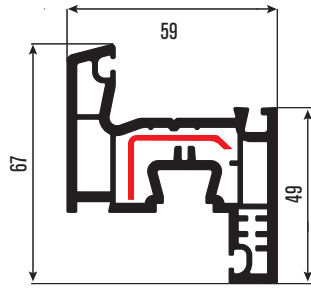
PRLT02 Kanat Profili Sash Profile DS-13
