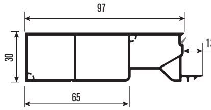
PRP741 Dış Parapet Uzun Profil Long Profile Of The Outer Parapet
