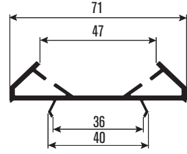
PR7127 Köşe Dönüş Adaptörü Adaptor To Turn Corner
