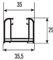
PRPJ87 29 mm Yan Dikme 29 mm Edge Pillar
