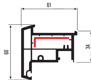
PR6013 Hareketli Orta Kayıt Stump (Overhang) DS-18
