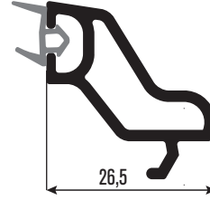
PR7120 24mm Dekoratif Cam Çıtası 24mm Decorative Glazing Bead
