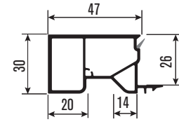
PRP740 Dış Parapet Kısa Profil Short Profile Of The Outer Parapet
