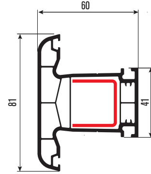
PRVN03 Orta Kayıt Profili Mullion Profile DS-2
