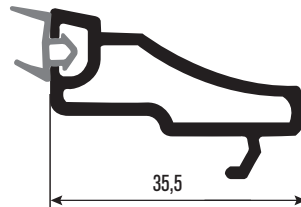
PR6015 Dekoratif Tek Cam Çıtası Decorative Single Glazing Bead
