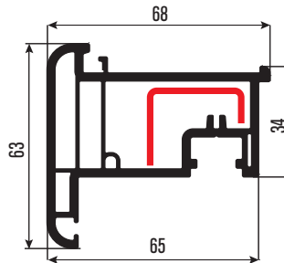
PR7113 Hareketli Orta Kayıt Stump (Overhang) DS-12
