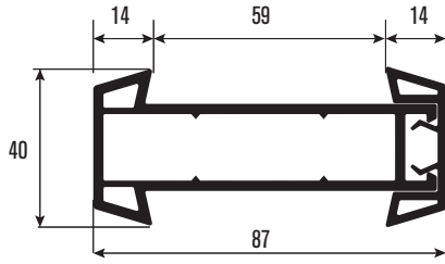
PR6025 Geniş Bağ Profili Profile of Wide Band
