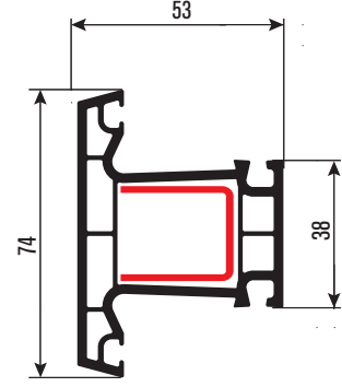
PRFS03 Orta Kayıt Profili Mullion Profile DS-03
