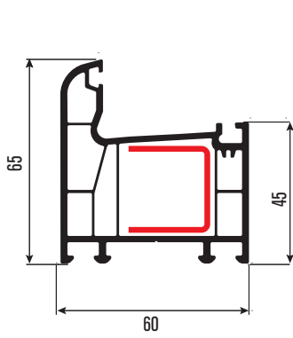
PRVN01 Kasa Profili Frame Profile DS-2
