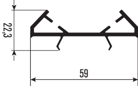
PR6027 Köşe Dönüş Adaptörü Adaptor To Turn Corner
