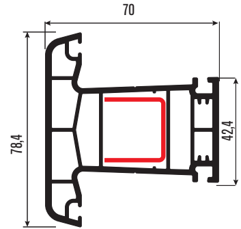
PRP703 Orta Kayıt Profili Mullion Profile DS-2
