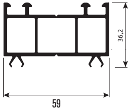
PR6037 Kasa Yükseltme Profili Frame Joint Profile
