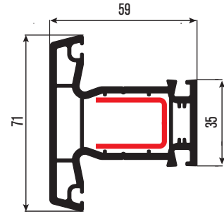
PRLT03 Orta Kayıt Profili Mullion Profile DS-3 DS-20
