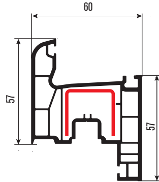
PRVN02 Kanat Profili Sash Profile DS-2
