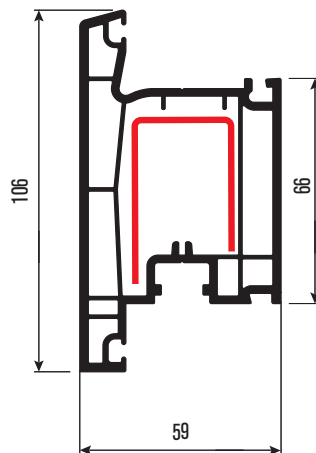
PR6005 Dışa Açılım Kapı Profili Outside Opening Door Sash Profile DS-28 DS-14
