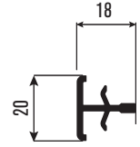
PRTS24 İnce Bağ Profili Coupling
