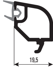
PRVN17 20mm Çift Cam Çıtası 20mm Double Glazing Bead
