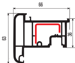
PRR713 Hareketli Orta Kayıt Stump (Overhang)
