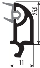
PRVN21 30mm Çift Cam Çıtası 30mm Glazing Bead
