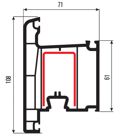
PR7105 Dışa Açılım Kapı Profili Outside Opening Door Profile DS-8 DS-14
